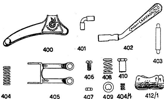
PARTICOLARI DEL 1011
